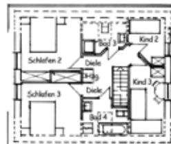
Dachgeschoss
